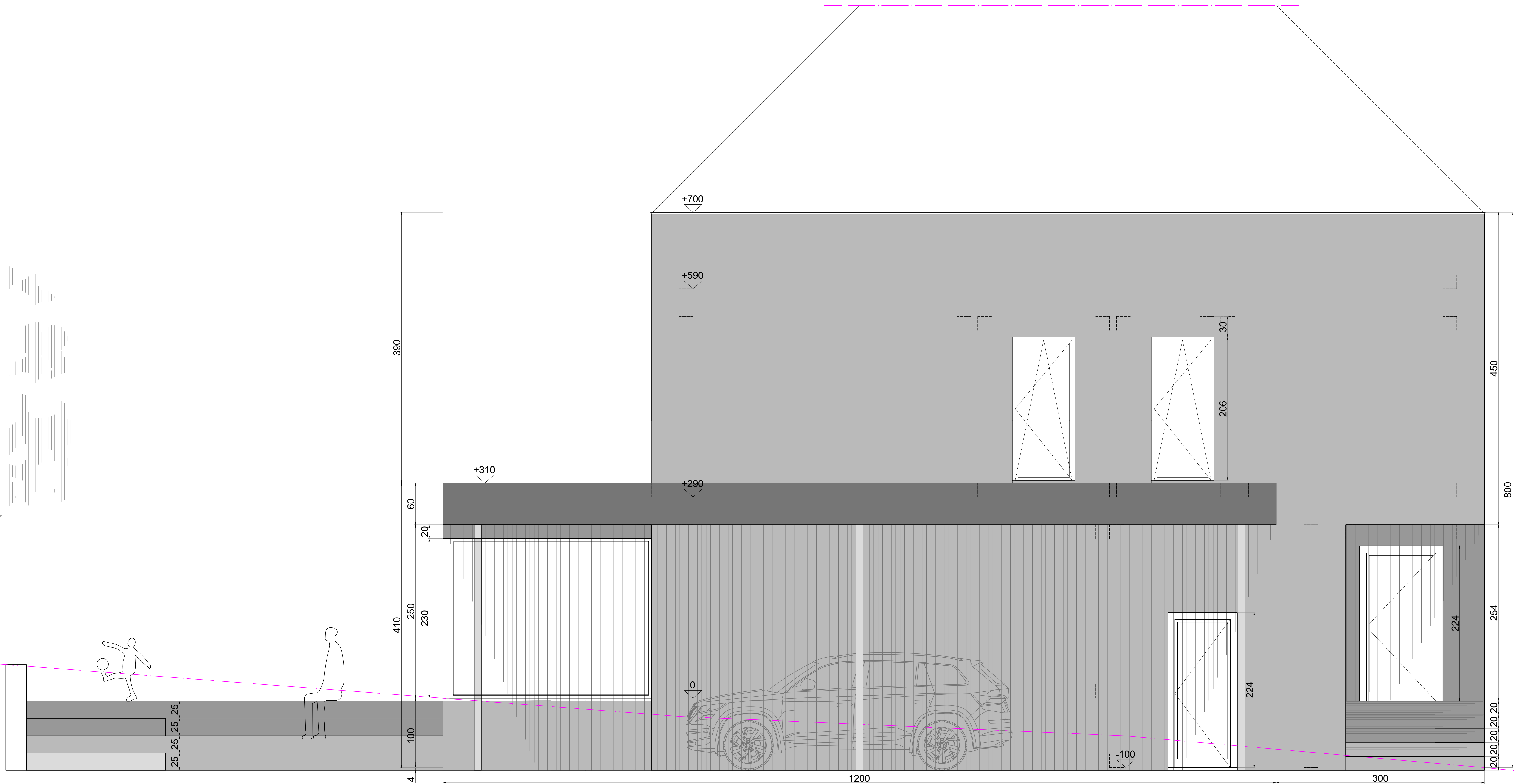
ZIJGEVEL LINKS
